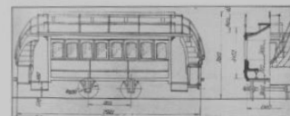
Чертежи вагонов Петербургской конно-железной дороги. Продольная разбивка вагонов вместимостью соответственно до 45, 51 и 77 человек.
