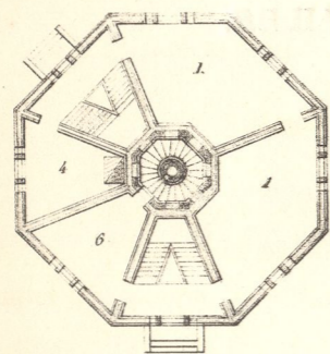
Планъ первого этажа
